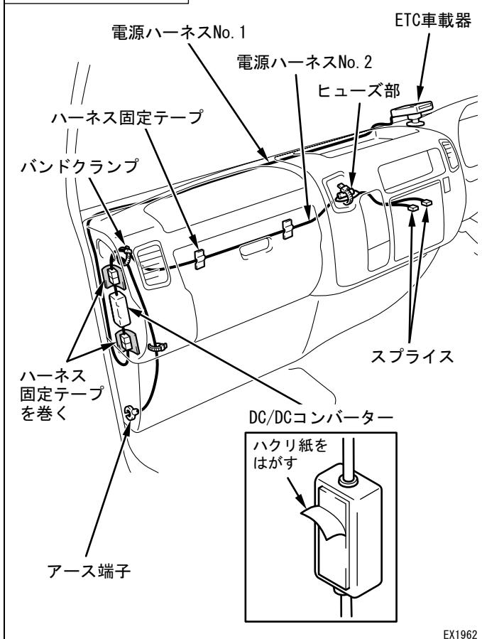
左側配線例 (24V車用)
