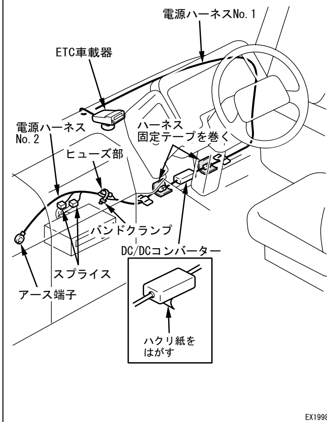
左側配線例 (24V車用)
