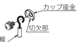
＜丸形圧着端子を使用しない場合＞
