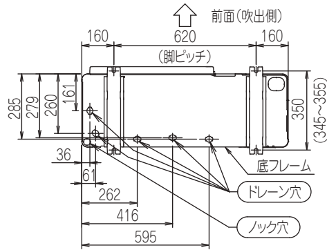
下面図(単位mm)
