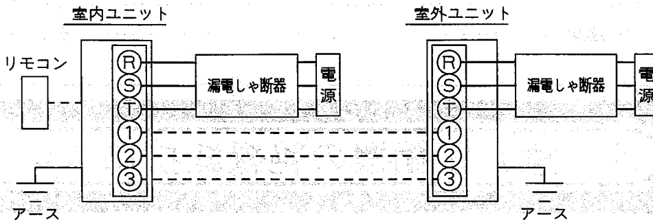
標準配線器具明細(内線規程JEAC8001)
